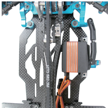
図① バッテリー横置きの場合
